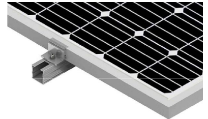
Détail fixation latérale
